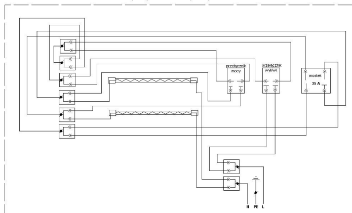
Schemat połączeń elektrycznych Wulkan 2500
